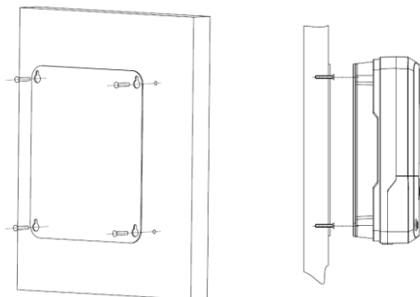
Рисунок 2.2. Последовательность монтажа
