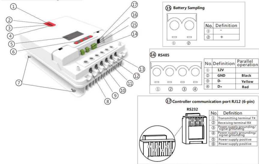
Рисунок 1-1. Внешний вид контроллера и разъемы
